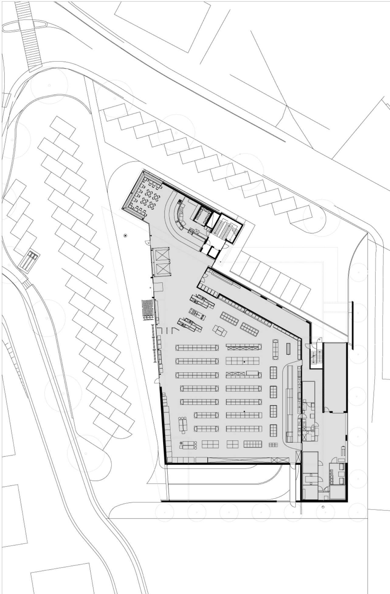
Grundriss Erdgeschoss
